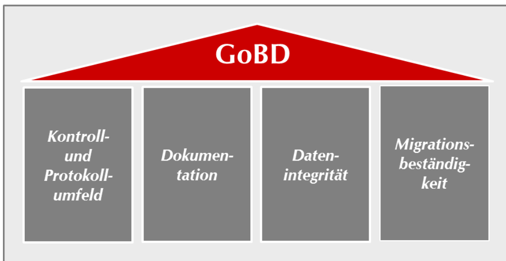
Abbildung: Vier-Säulen-Modell
